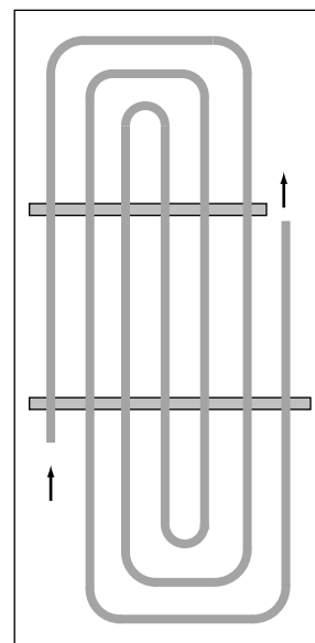
Draufsicht Wandheizungsregister
